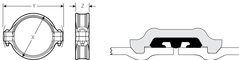
Typisk 14 – 24"/DN350 – DN600
