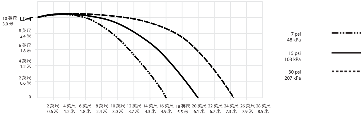
型号 V3409、V3410 K8.0 标准水平侧墙式及凹装水平侧墙式分布模型 - 曲线图
