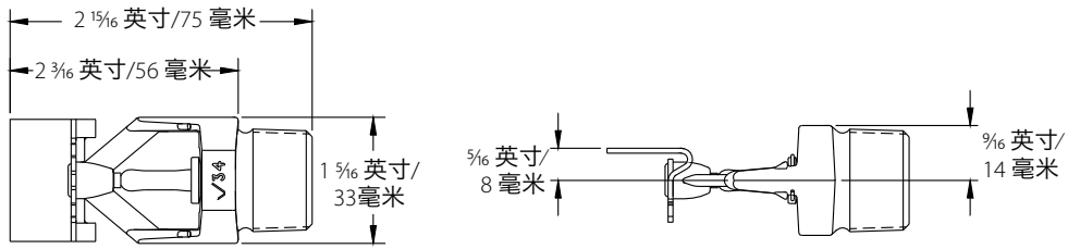
标准水平侧墙式 - V3409、V3410
