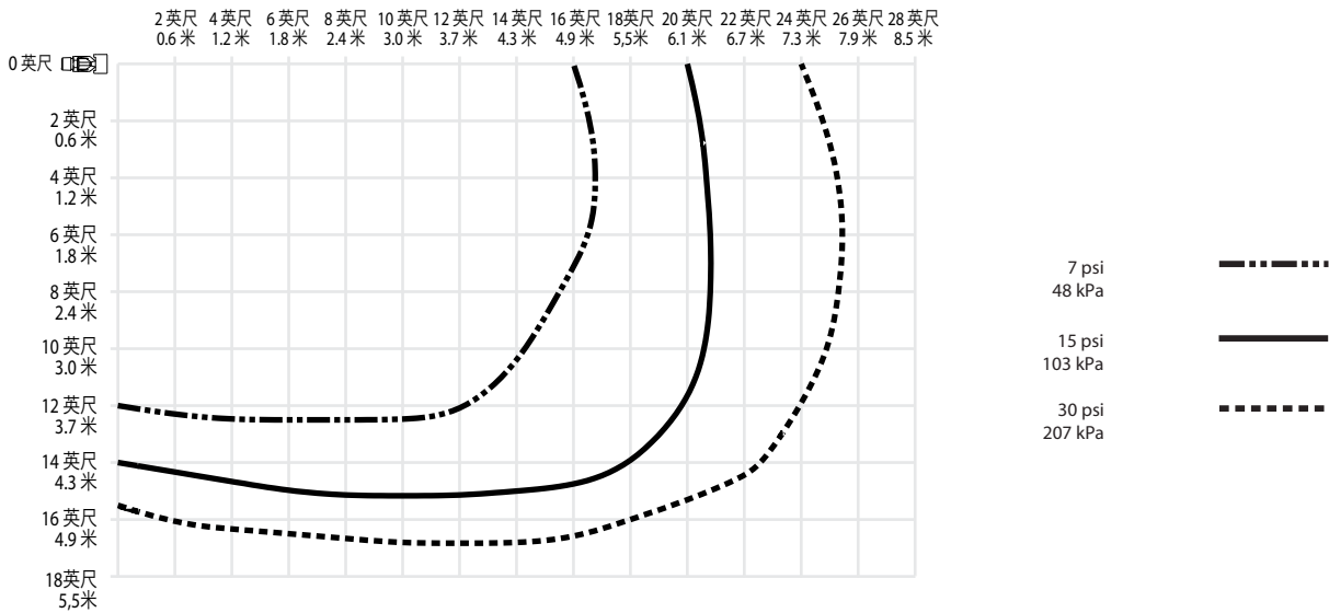
型号 V3409、V3410 K8.0 标准水平侧墙式及凹装水平侧墙式分布模型 - 平面图
