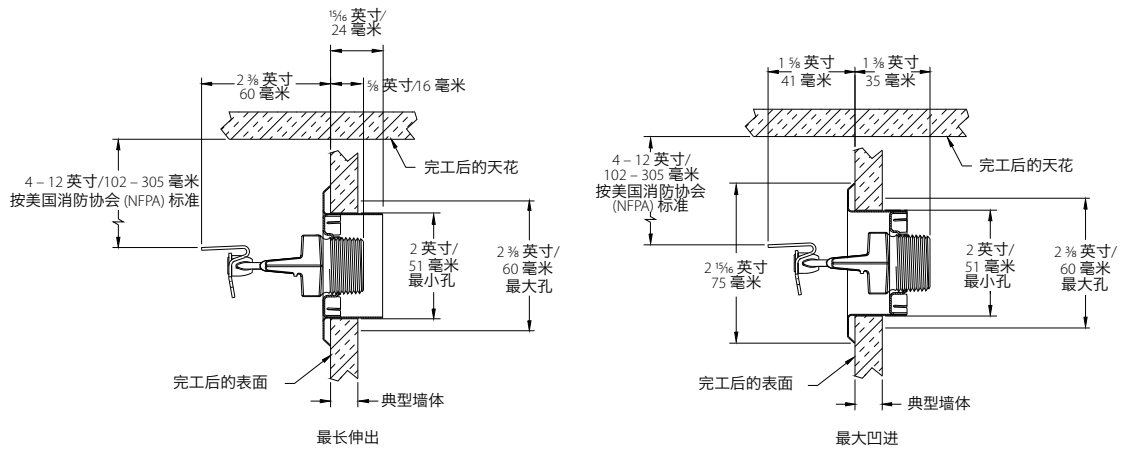
3/4 英寸调节量凹装式 - V3409、V3410 (图不是按比例画出)
