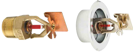
水平侧墙式 (V3409 和 V3410)
