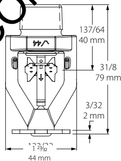
标准下喷式 V4402
